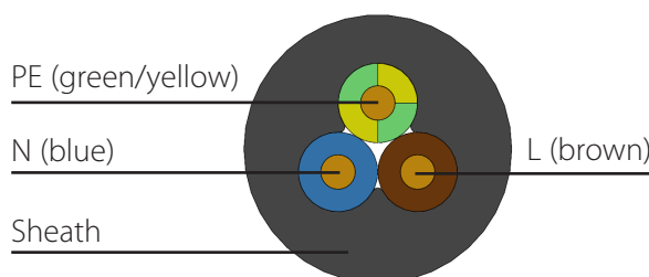
AC input
