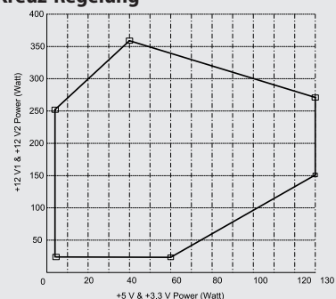
Kreuz-Regelung
